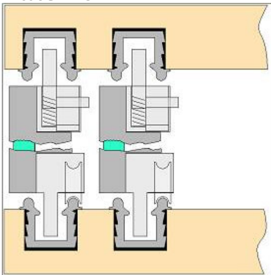
Einbauskizze
