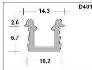
Querschnitt
